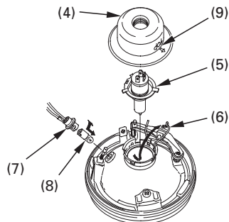
(4) Kumi (5) Ajovalopolttimo (6) Kiinnike
