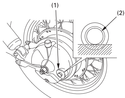
(1) Öljyn täyttölppa (2) Öljyn täyttöaukko
