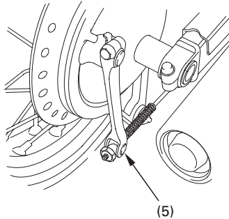
(5) Jarruvivun tappi
