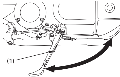
(1) Sivuseisontatuen jousi
